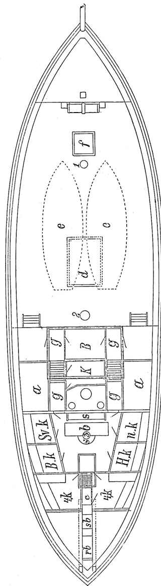
Fig. 2. Plan.
