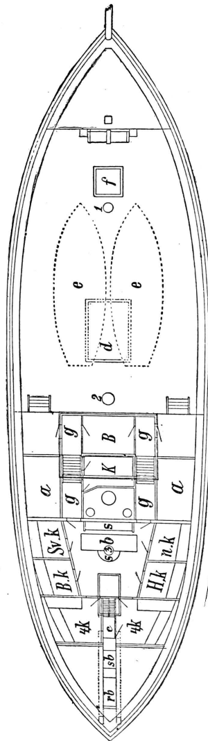
Fig. 2. Plan.
