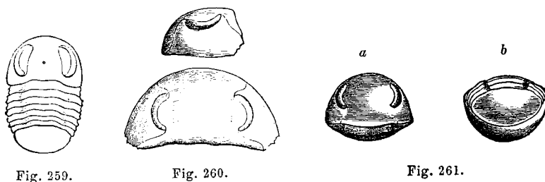
Fig. 259.— Nileus macrops .
