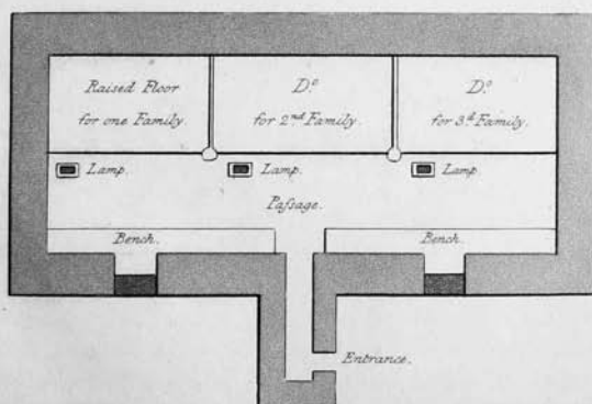
Ground-plan.
