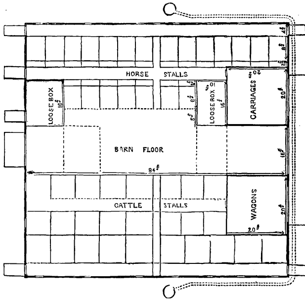
Fig. 15.—PLAN OF BARN.
