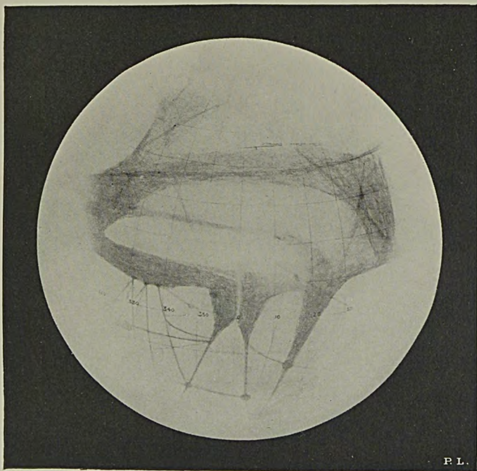
MARS LONGITUDE 0^{\circ} ON THE MERIDIAN
