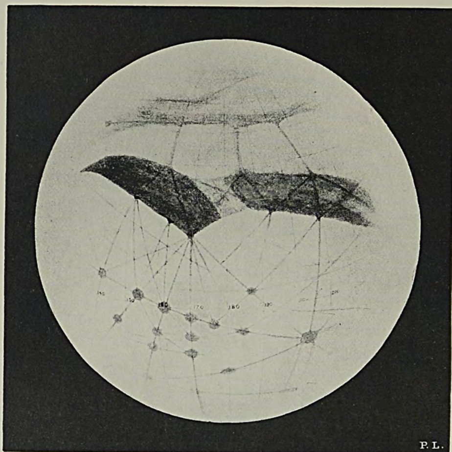
MARS LONGITUDE 180^{\circ} ON THE MERIDIAN
