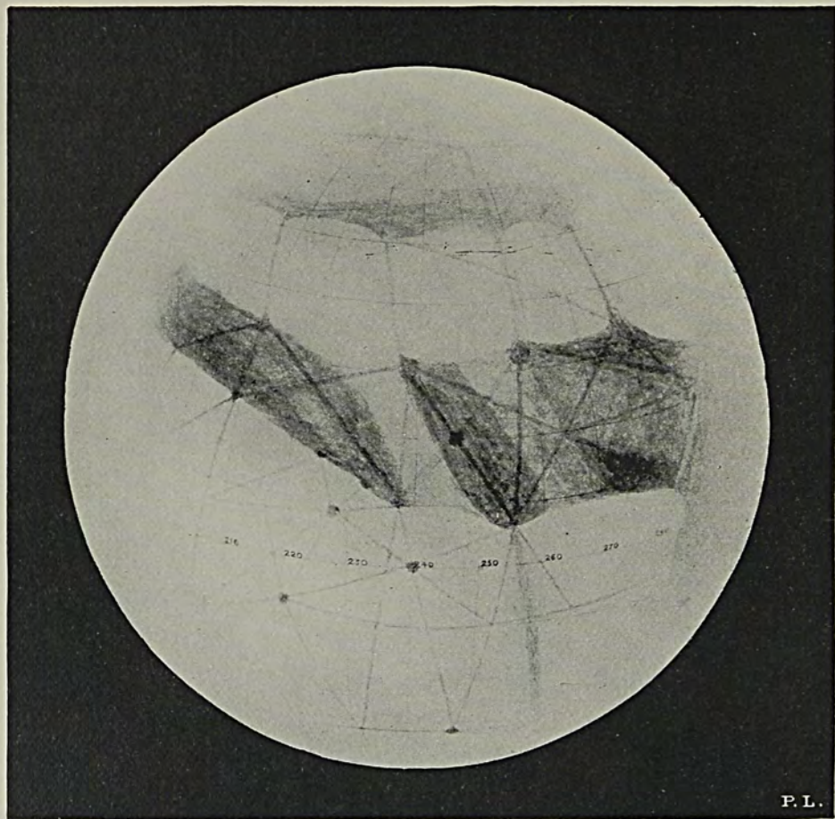
MARS LONGITUDE 240° ON THE MERIDIAN
