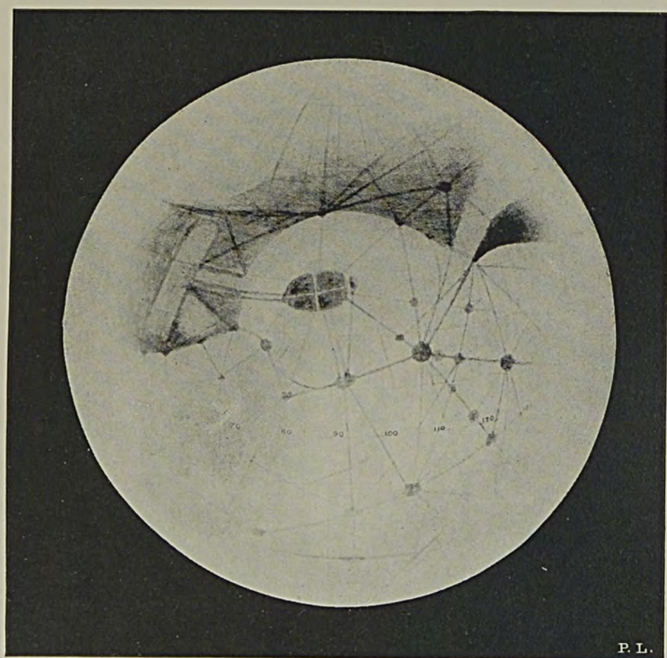
MARS LONGITUDE 90^{\circ} ON THE MERIDIAN
