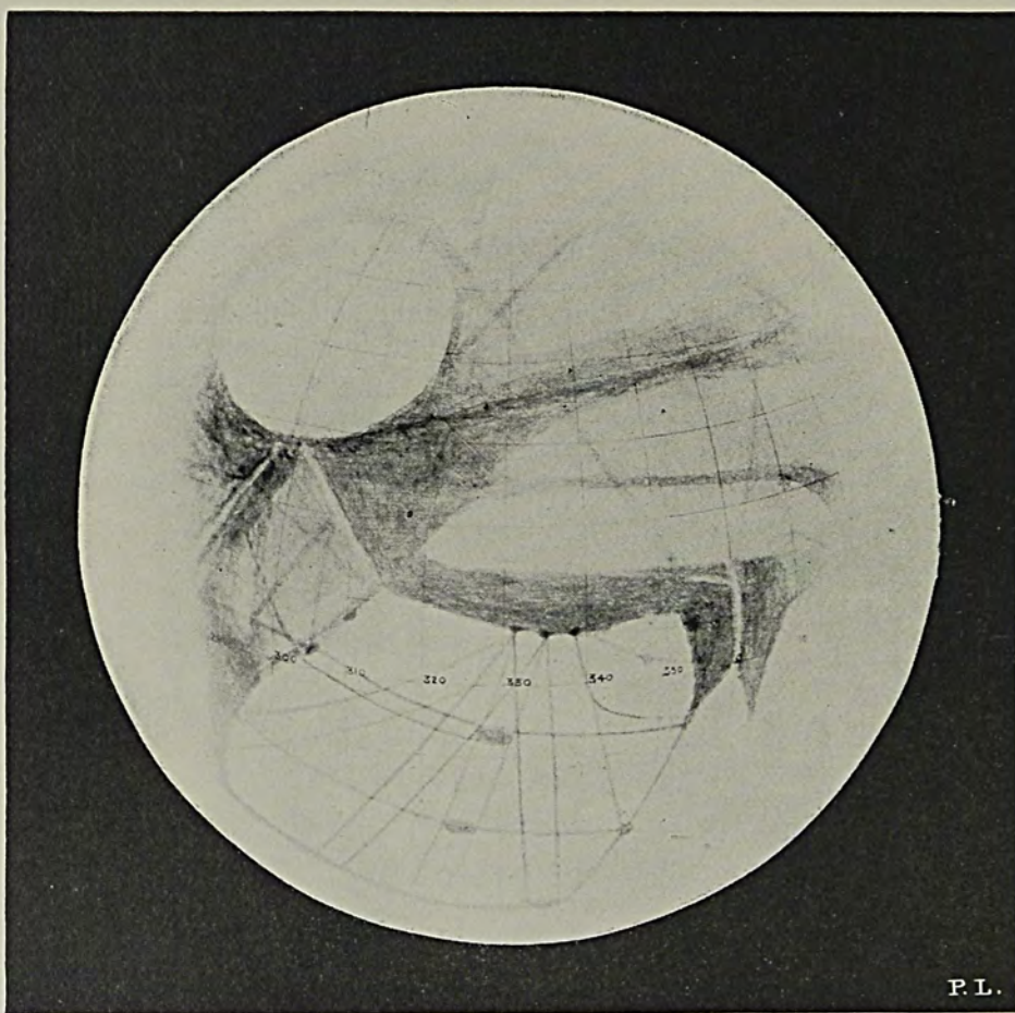
MARS LONGITUDE 330^{\circ} ON THE MERIDIAN
