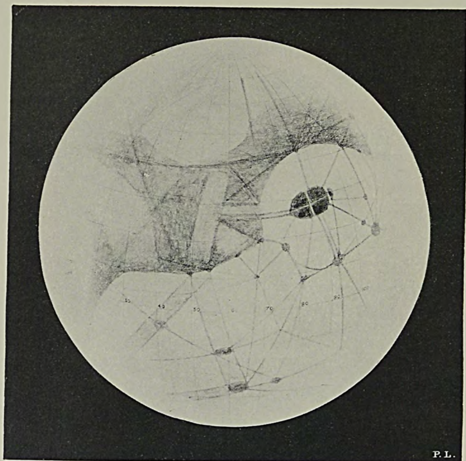
MARS LONGITUDE 60^{\circ} ON THE MERIDIAN
