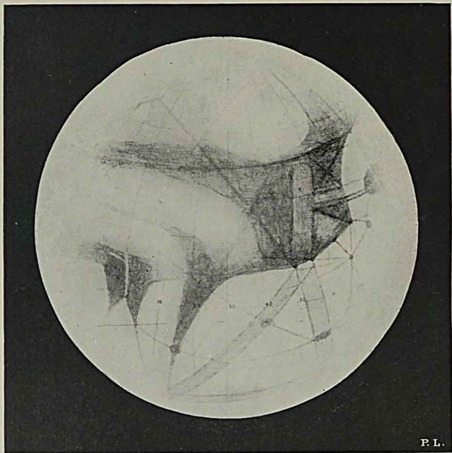
MARS LONGITUDE 30^{\circ} ON THE MERIDIAN
