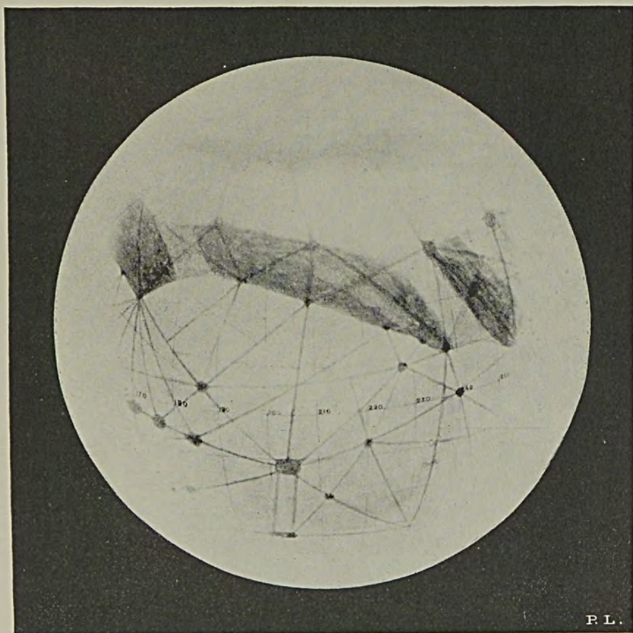
MARS LONGITUDE 210^{\circ} ON THE MERIDIAN
