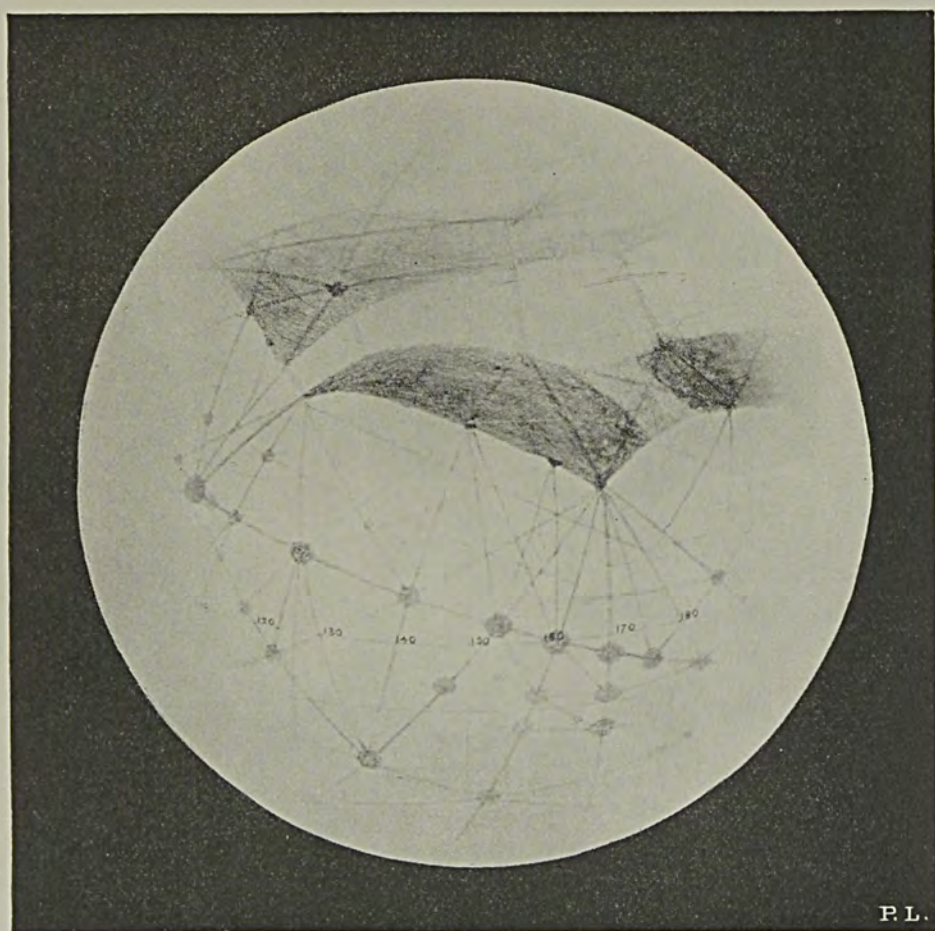
MARS LONGITUDE 150^{\circ} ON THE MERIDIAN
