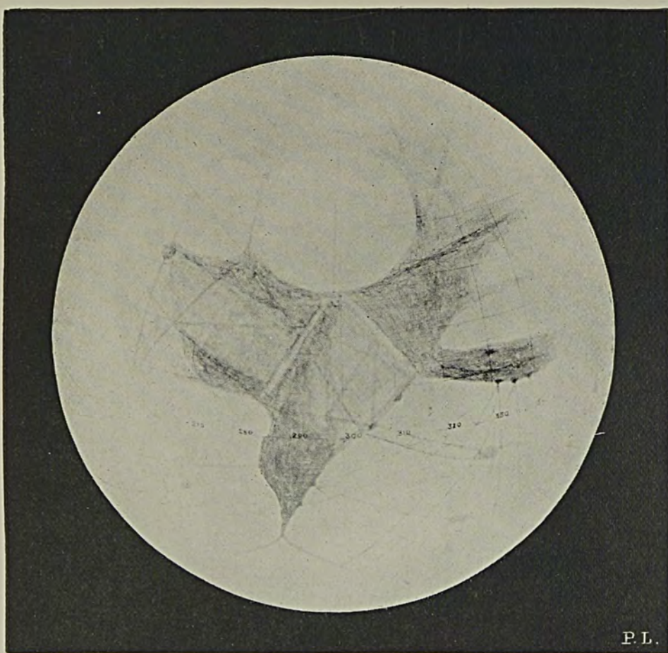
MARS LONGITUDE 300^{\circ} ON THE MERIDIAN
