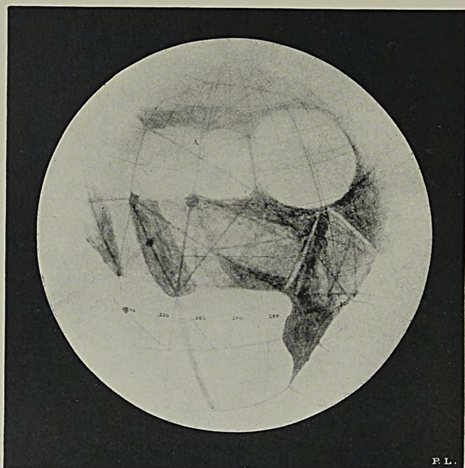
MARS LONGITUDE 270^{\circ} ON THE MERIDIAN
